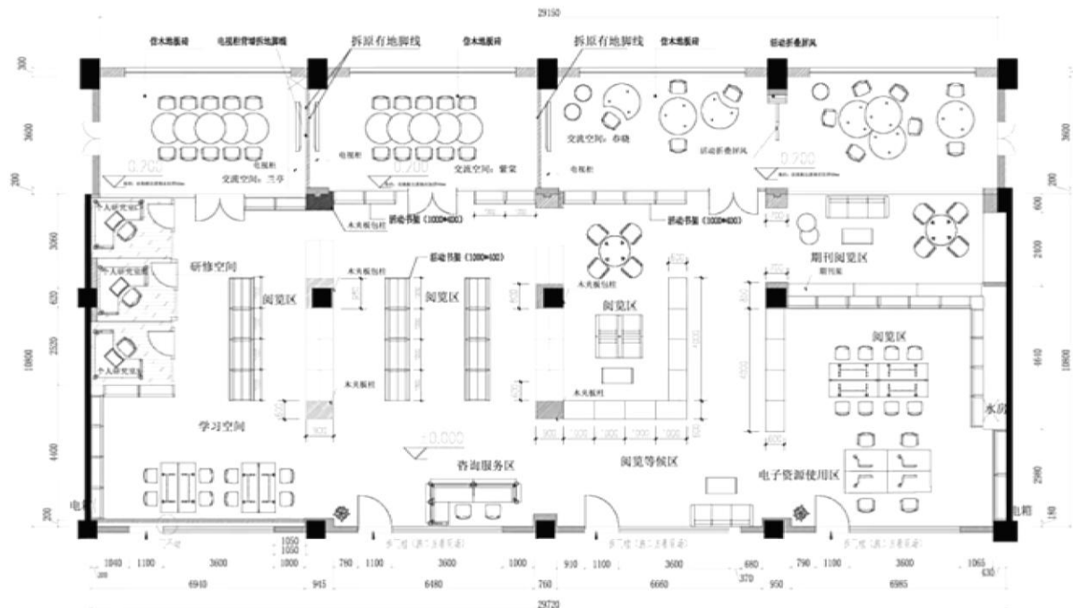
艺术专题共享空间平面布置图
